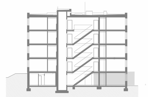
SVISLÝ ŘEZ
