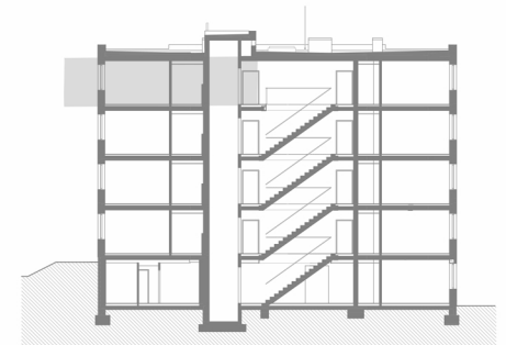
SVISLÝ ŘEZ
