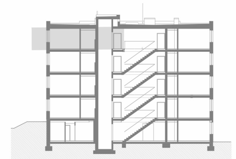
SVISLÝ ŘEZ
