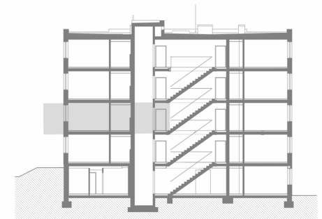
SVISLÝ ŘEZ
