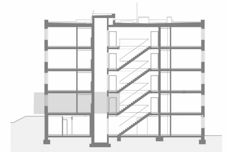
SVISLÝ ŘEZ
