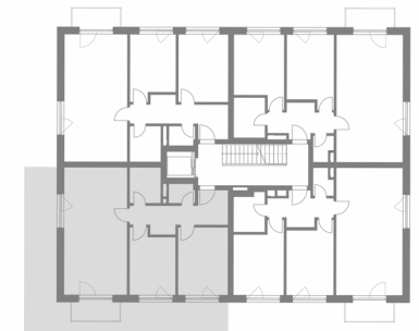
PŮDORYS 1.NP
