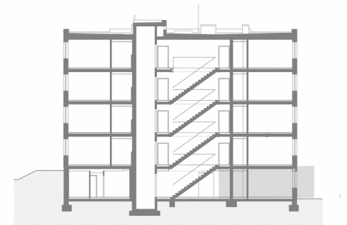
SVISLÝ ŘEZ
