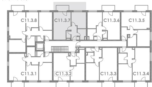
PŮDORYS 3.NP
