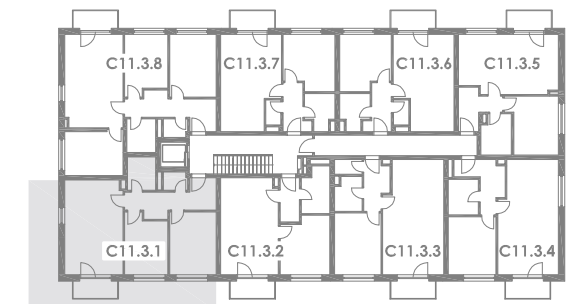
PŮDORYS 3.NP
