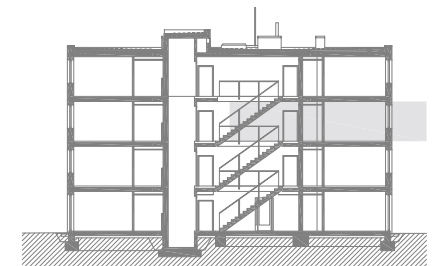
SVISLÝ ŘEZ
