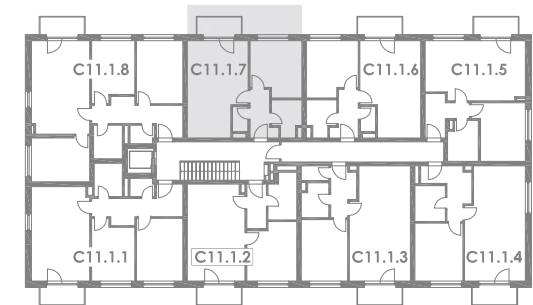
PŮDORYS 2.NP
